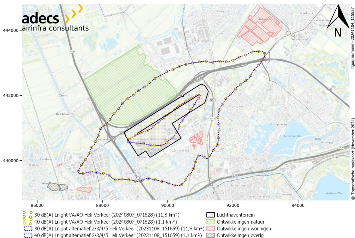
Figuur 48 Vergelijking van de 30 en 40 dB(A) L night -contouren van alle alternatieven voor het helikopterterverkeer.
