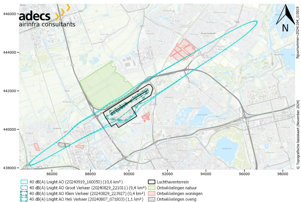
Figuur 43 40 dB(A) Night-contouren van de referentiesituatie in zichtjaar 2035 (autonome ontwikkeling) voor groot verkeer, klein verkeer en helikopterverkeer apart en gezamenlijk.
