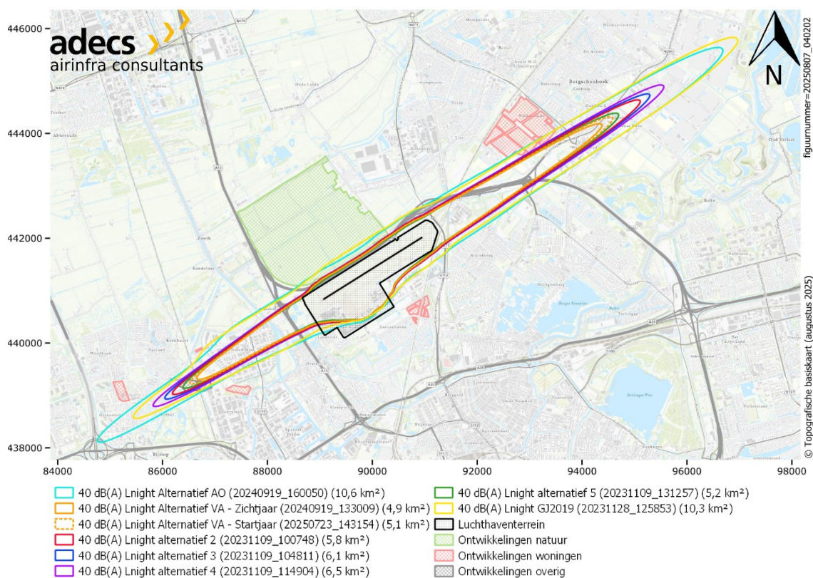
Figuur 33 Vergelijking van 40 dB(A) L_{night} -contouren van alle alternatieven.
