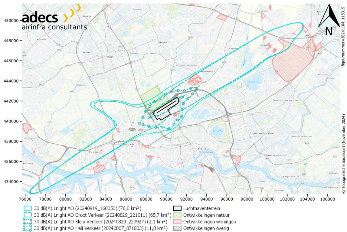
Figuur 44 30 dB(A) Night-contouren van de referentiesituatie in zichtjaar 2035 (autonome ontwikkeling) voor groot verkeer, klein verkeer en helikopterverkeer apart en gezamenlijk.
