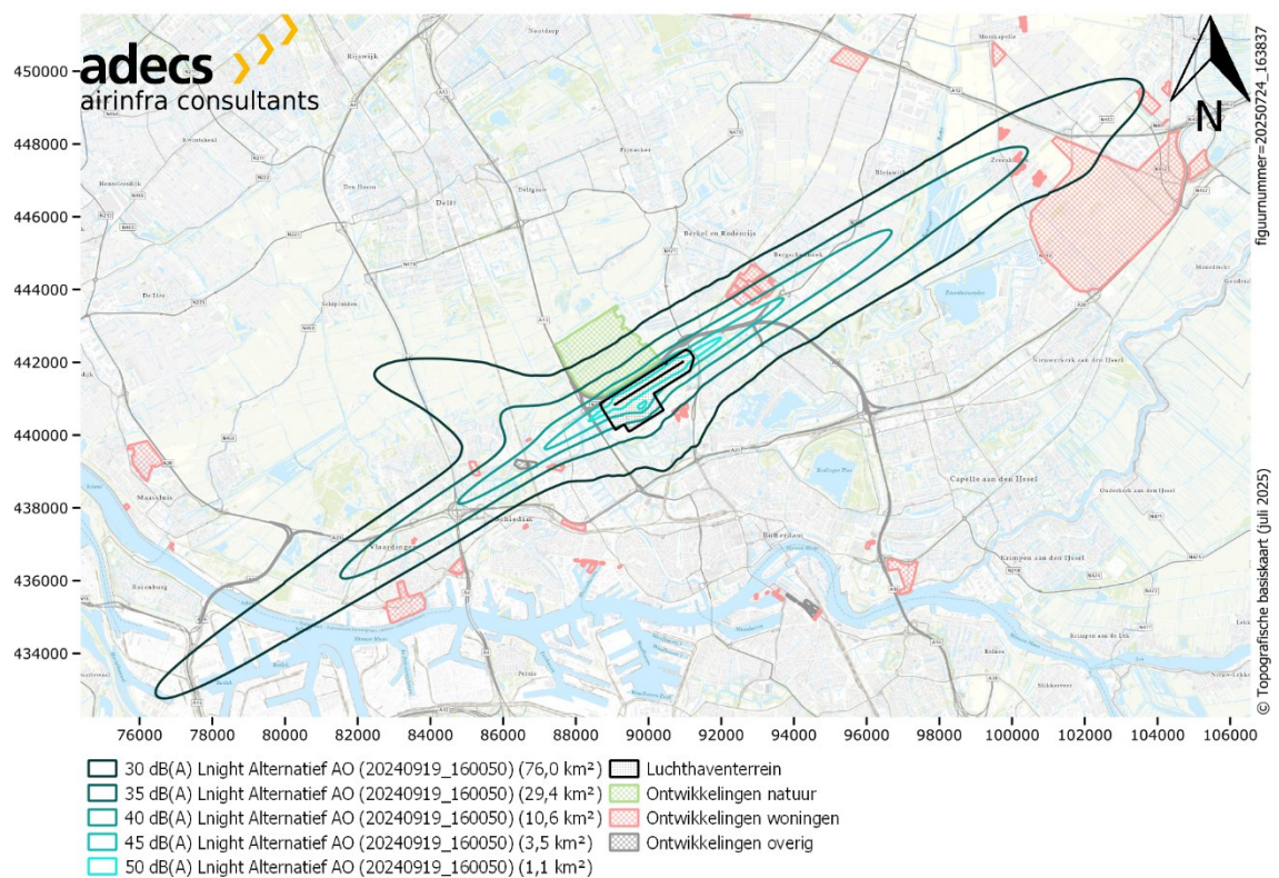
Figuur 31 30, 35, 40, 45 en 50 dB(A) L night -contouren van de referentiesituatie in zichtjaar 2035 (autonome ontwikkeling).
