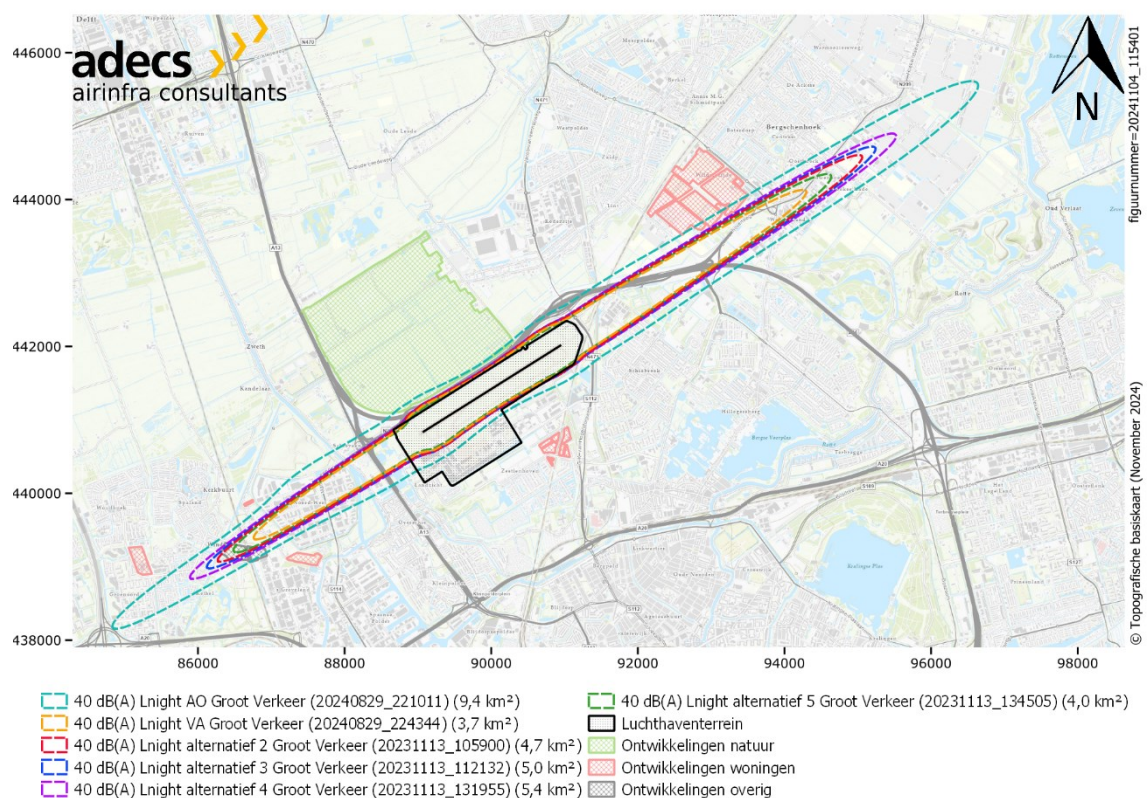
Figuur 45 Vergelijking van 40 dB(A) L_{night} -contouren van alle alternatieven voor het groot verkeer.
