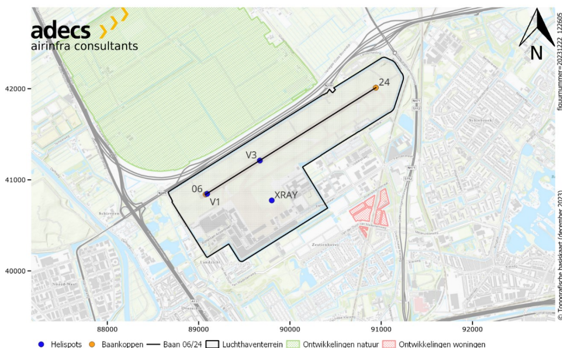
Figuur 12 Geografische ligging van de baankoppen en de helispots.
